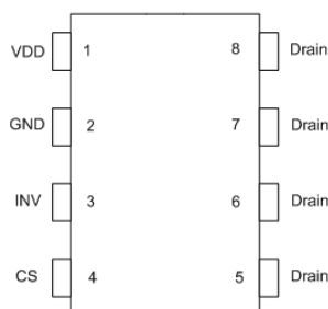
SOP8
